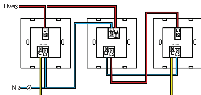
Междинен - триполюсен
